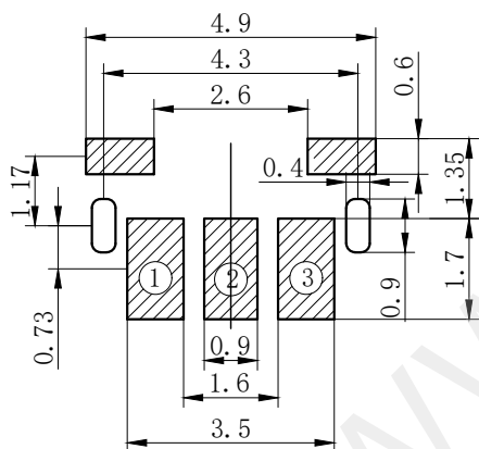
安装参考图
